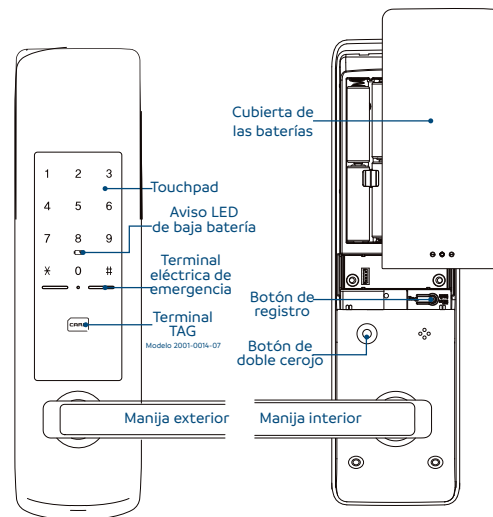
Cuerpo externo
